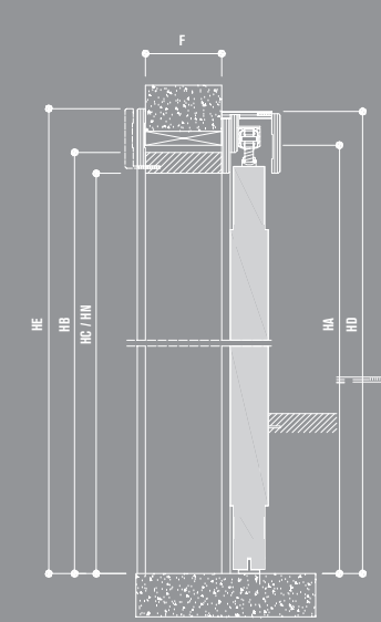
Porta Scorrevole esterno muro Sliding door
