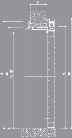
Porta Scorrevole esterno muro Sliding door
