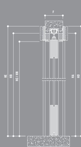
Porta Scorrevole interno muro Hidden Sliding door
