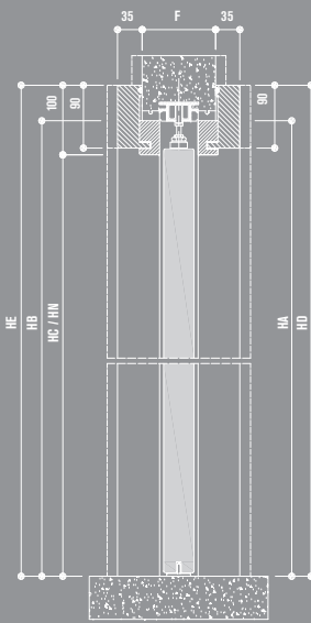
Porta Scorrevole interno muro / Hidden Sliding door
