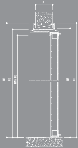
Porta Battente / Hinged door
