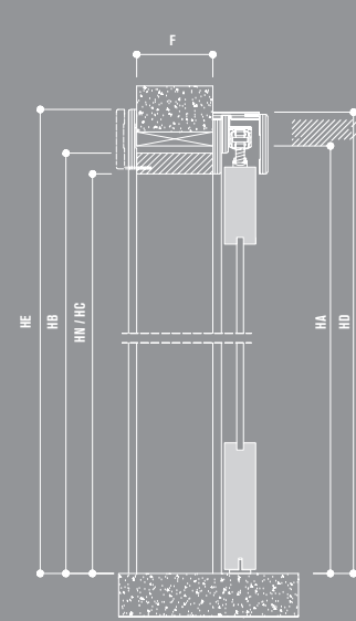
Porta Scorrevole esterno muro Sliding door
