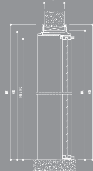
Porta Battente / Hinged door
