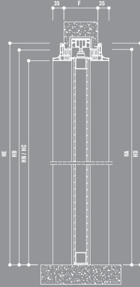
Porta Scorrevole interno muro Hidden Sliding door
