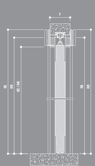
Porta Scorrevole interno muro Hidden Sliding door
