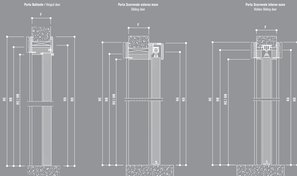
Porta Battente / Hinged door
