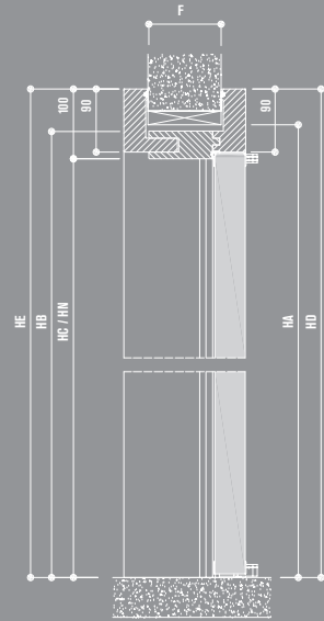
Porta Battente / Hinged door
